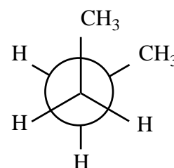
Gauche
