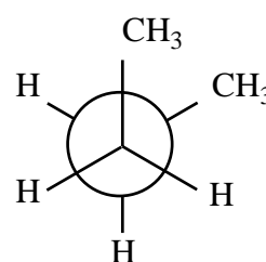
Gauche
